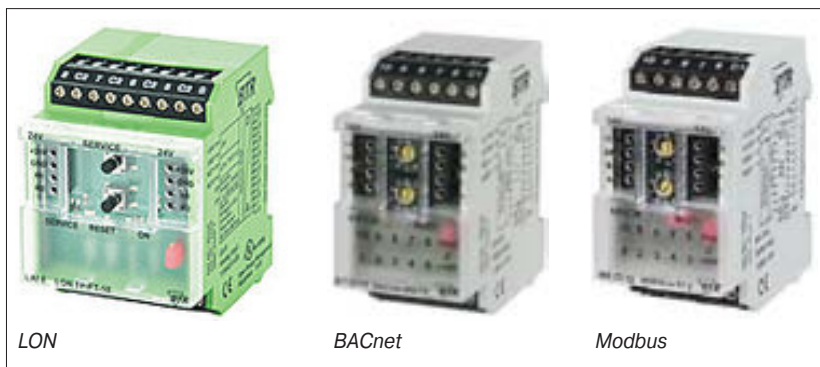
Модули ввода/вывода Logline
