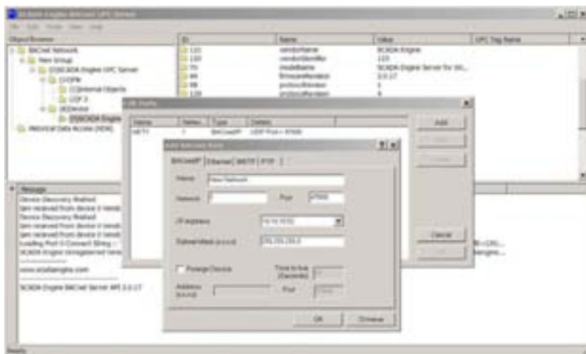
Интерфейс SE-OPC для сетей VACnet
